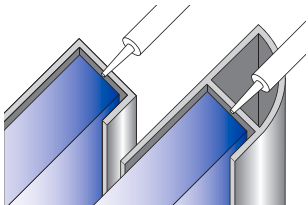
End Cap / End Cap Quad
