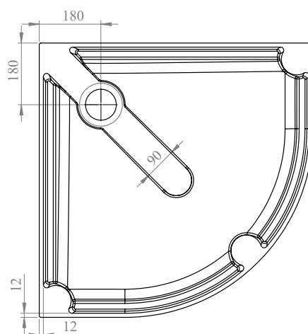
PRZEKRÓJ M-M SKALA 1 : 10
