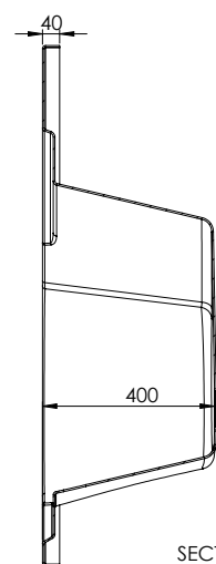
SECTION N-N SCALE 1 : 10
