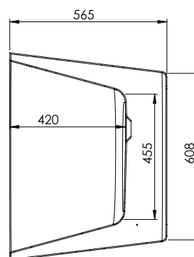
SECTION J-J SCALE 1 : 10
